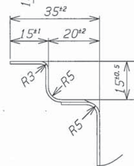
A-A' 断面 S=1/1
