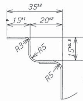
B-B' 断面 S=1/1
