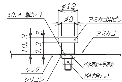
アミカゴ用ピン取付詳細 S=1/1
