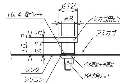
アミカゴ用ピン取付詳細 S=1/1
