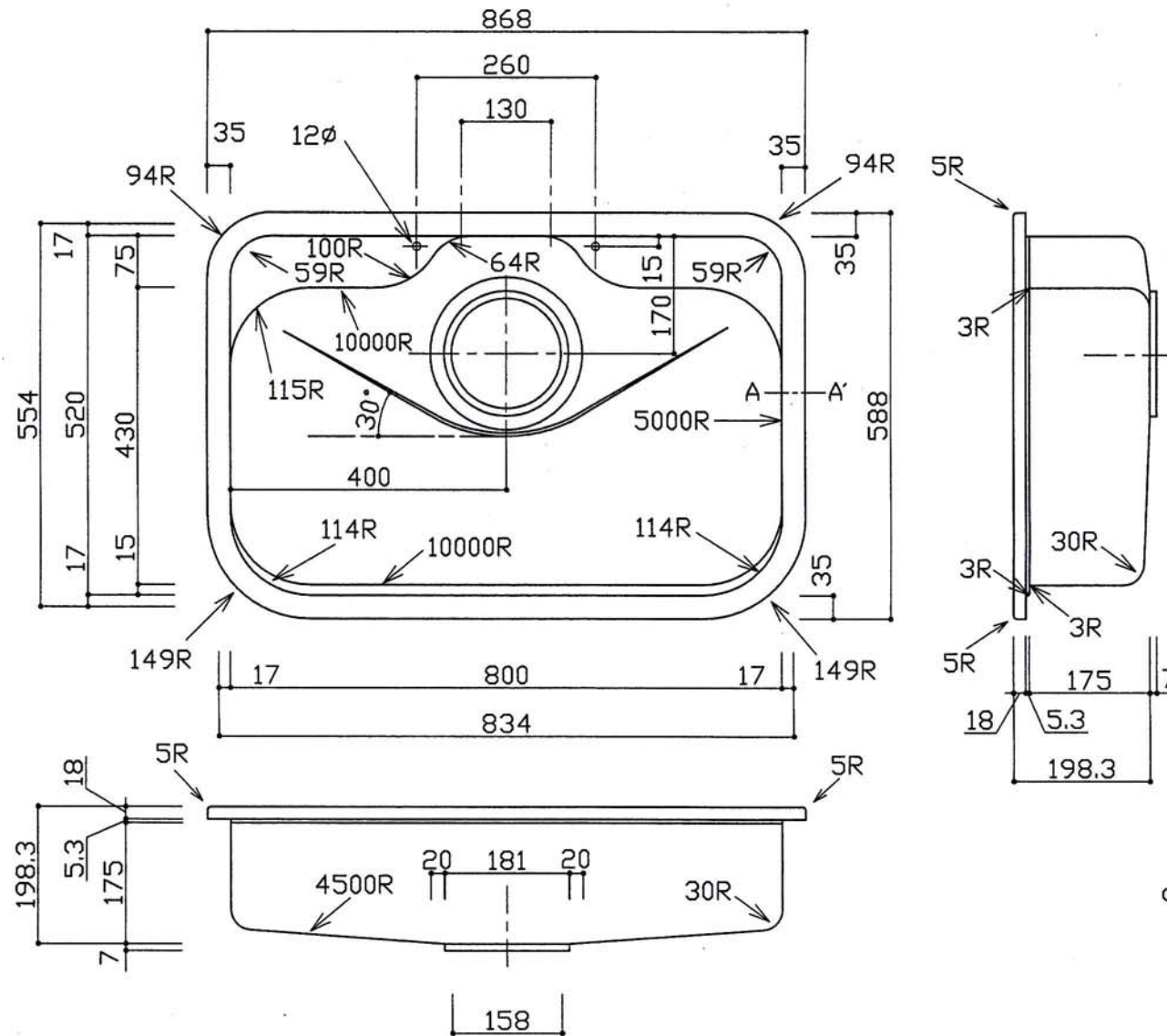
A-A' 断面詳細図
